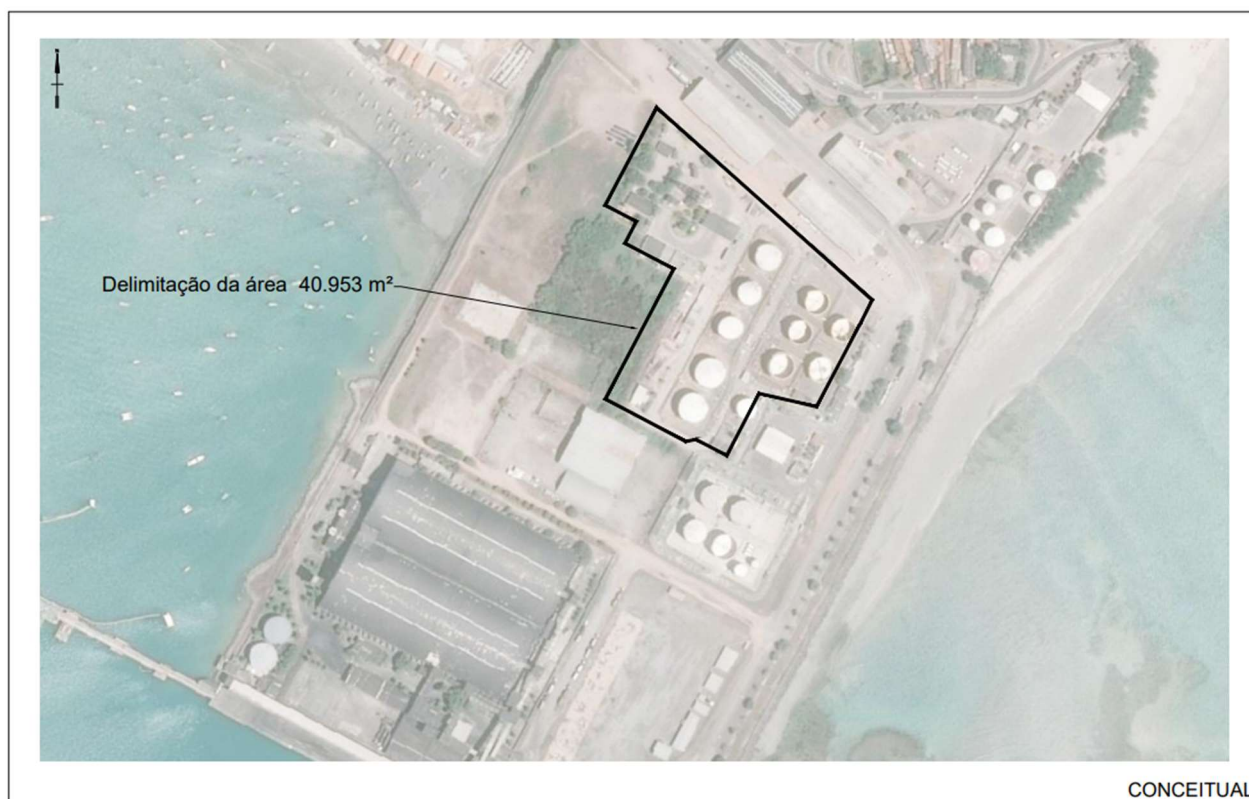
Figura 1: Layout geral da área de arrendamento MAC11A – Porto de Maceió.
